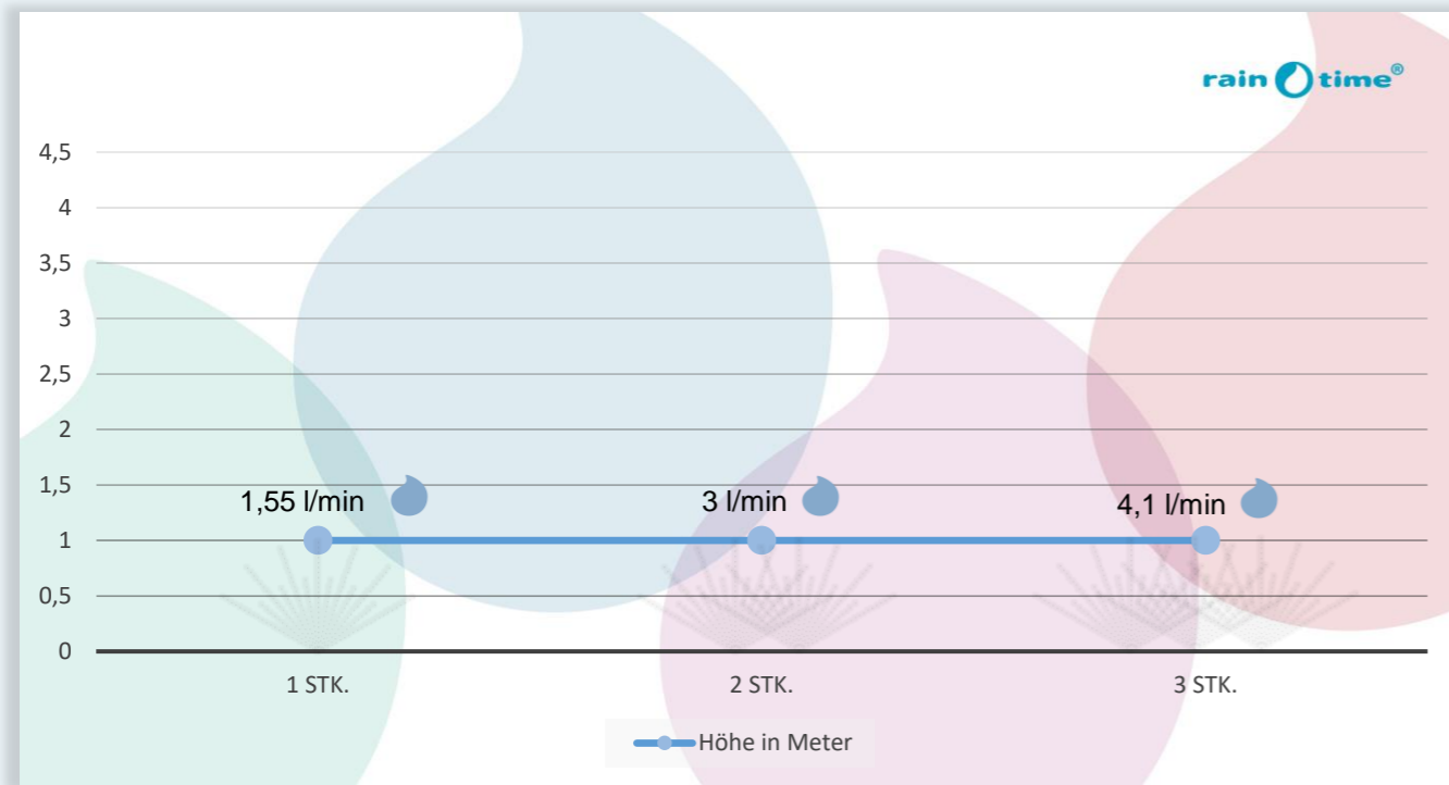
Verbrauch von 1 bis 3 Sprühdüsen (l/min) bei einer Höhe von 1 Meter
