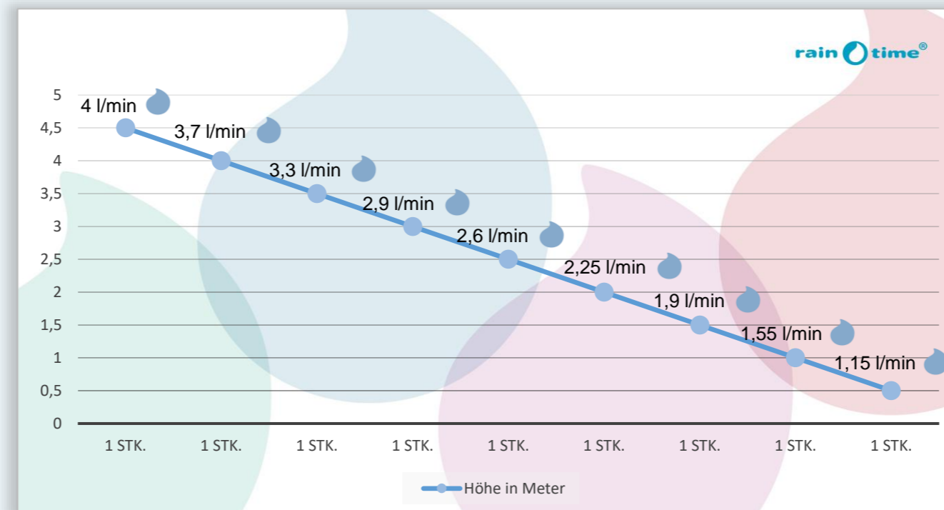
Verbrauch einer Sprühdüse (l/min) in Abhängigkeit von der Höhe
