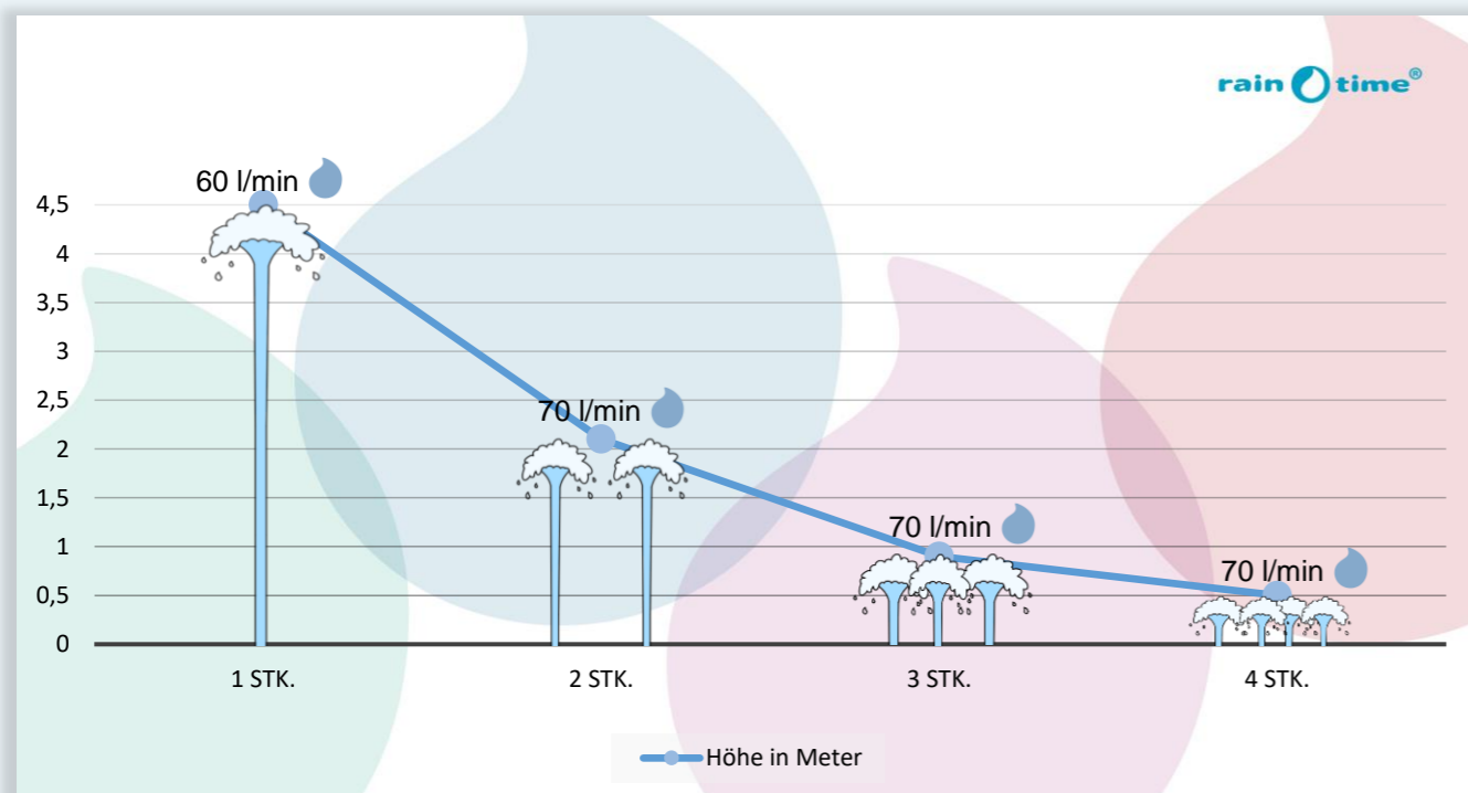
Verhalten der Fontänenhöhe bei vollständiger Auslastung der Pumpe mit maximal 4,2 bar, etwa 70 l/min
